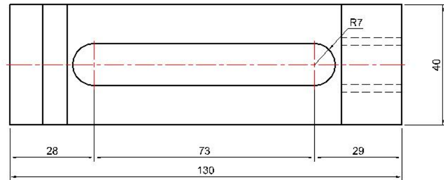
VISTA SUPERIOR
