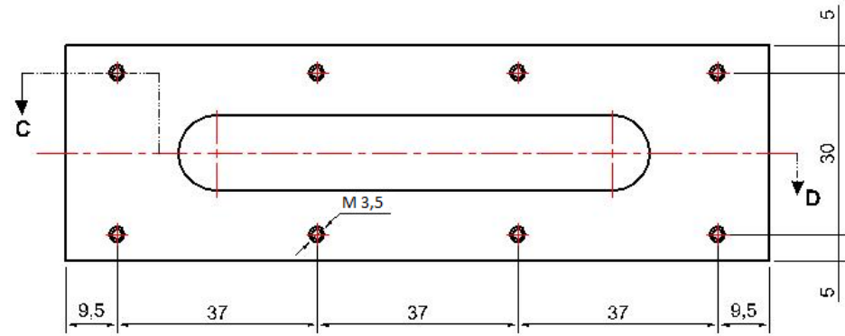
VISTA A
