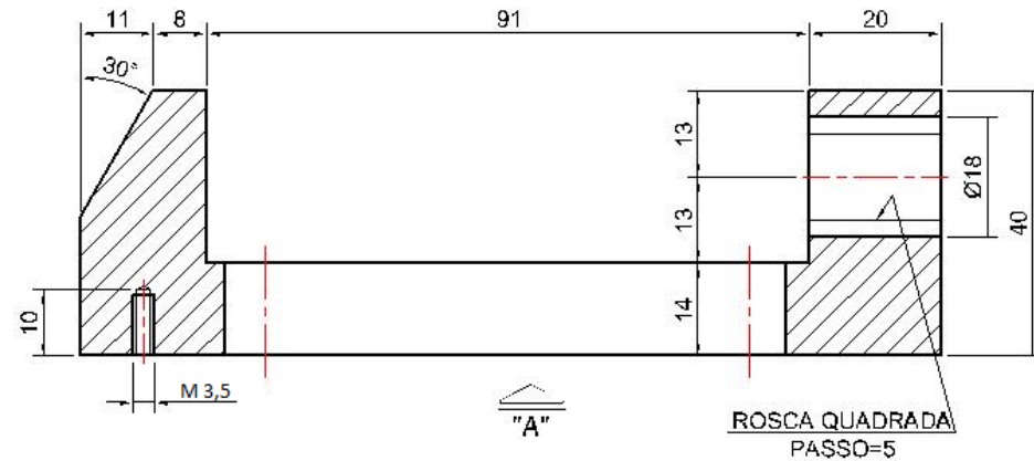
CORTE CD
