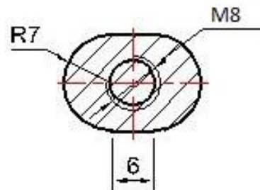
CORTE AB
