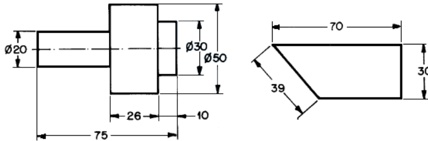
Figura – Localização das cotas no método 2
