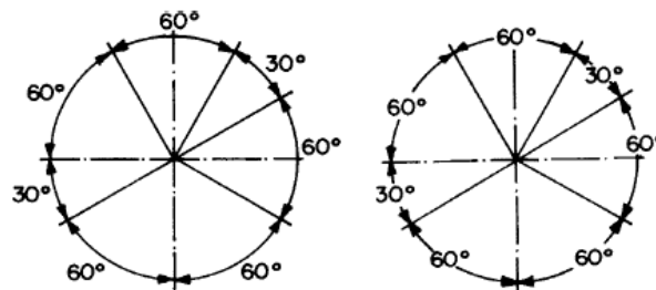
Figura – Cotagem angular no método 2
