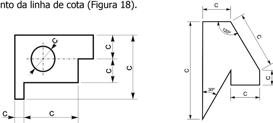
Figura 18 – Exemplos de cotação
