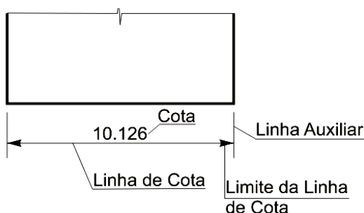
Figura 17 – Elementos de cotação
